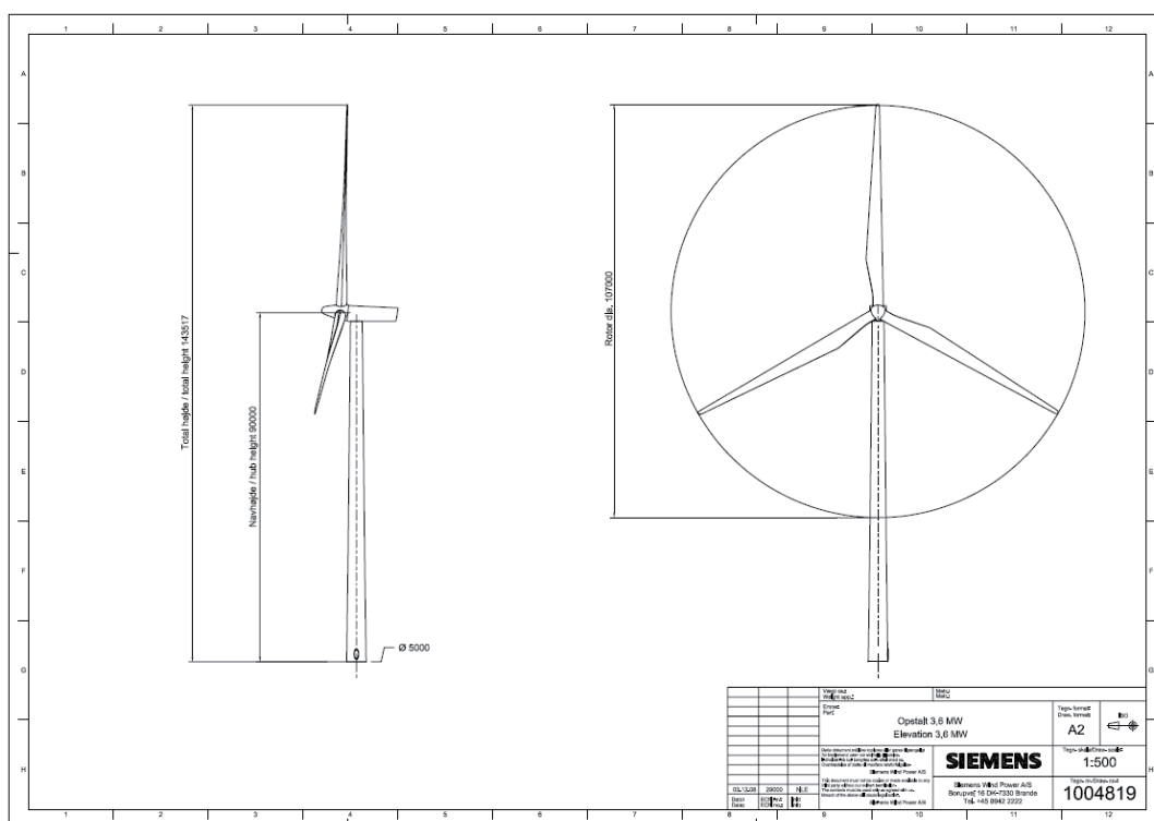
Kuva 1. Yleiskuva tuulivoimayksikön rakenteesta.
