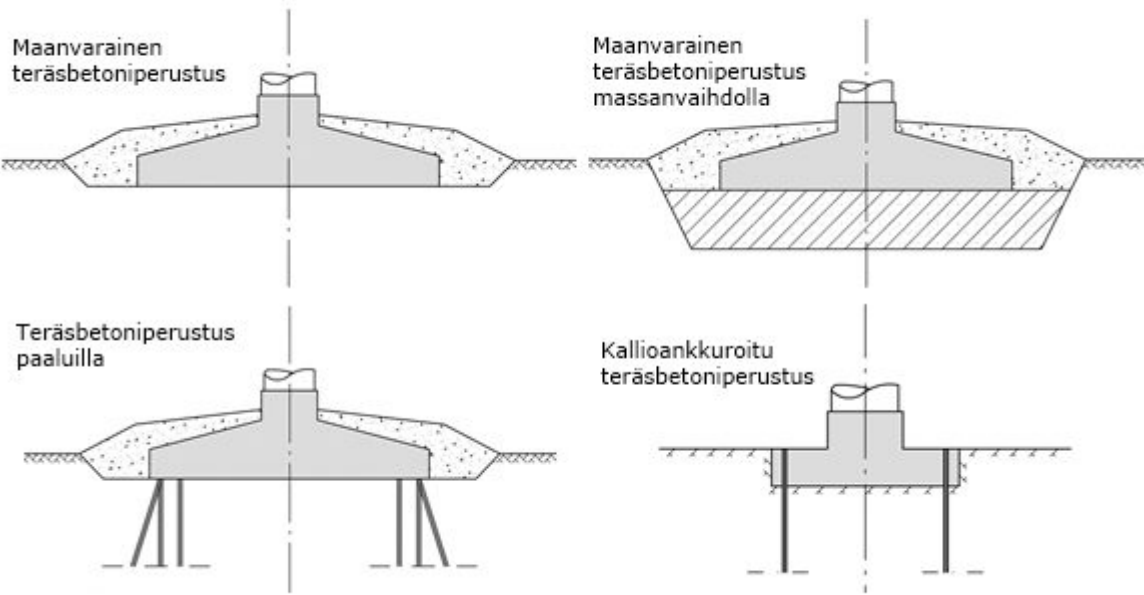
Kuva 8. Tuulivoimalaitosten perustamistekniikoita.
